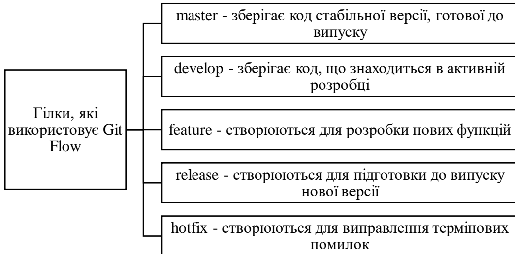
Рис. 1. Гілки Git Flow
