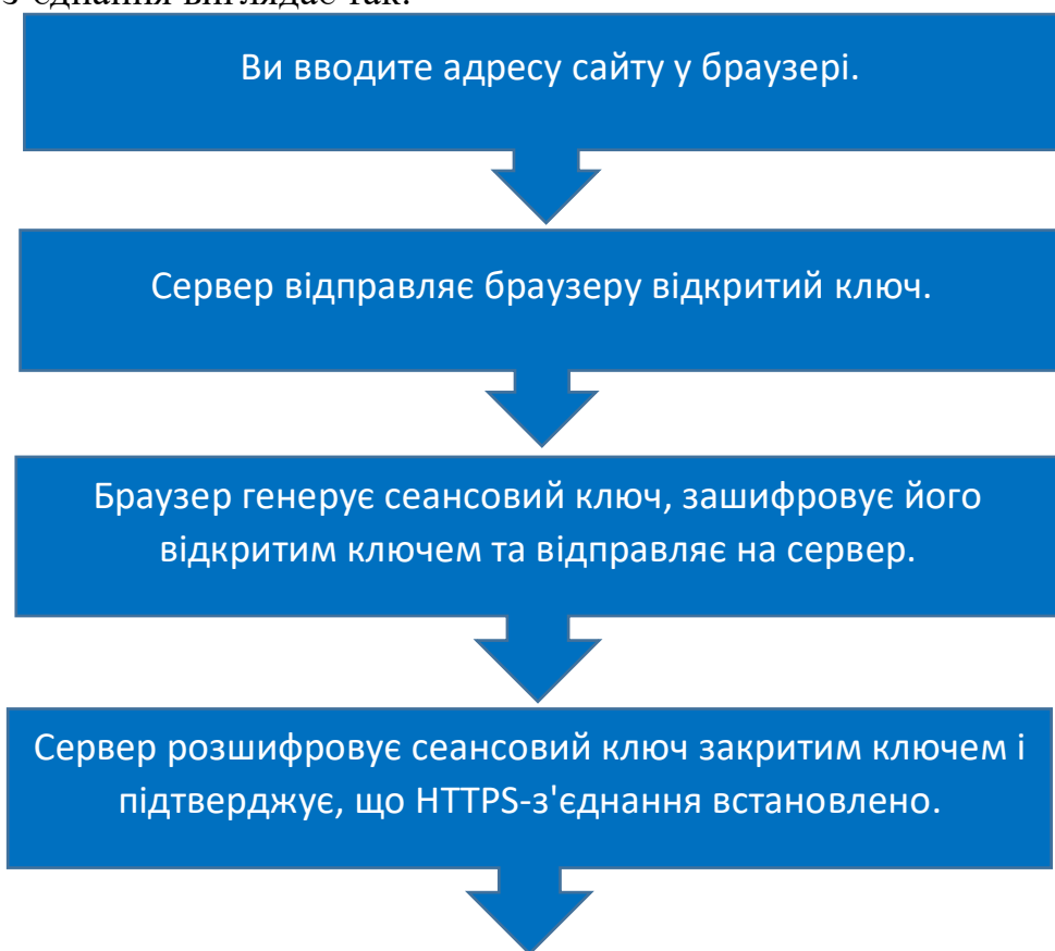
Рис. 1. Схематичне встановлення безпечного з'єднання
