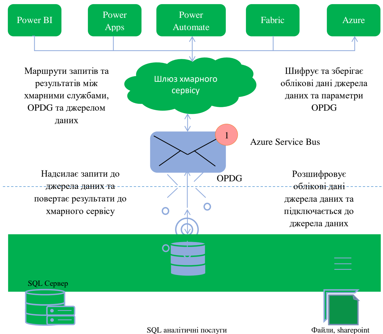
Рис. 1. Як працює On-Premise Data Gateway
